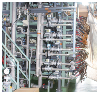
改良予定の脱臭塔（右）、膜分離装置（左）
