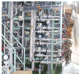
改良予定の脱臭塔(右)、膜分離装置(左)
