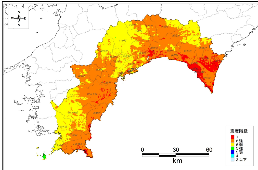
■ 震度分布図（詳細震度分布）
