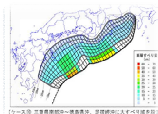
【ケース② 三重県南部沖～徳島県沖、足摺岬沖に大すべり域を設定】
