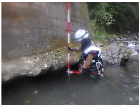
●下部工の洗掘
