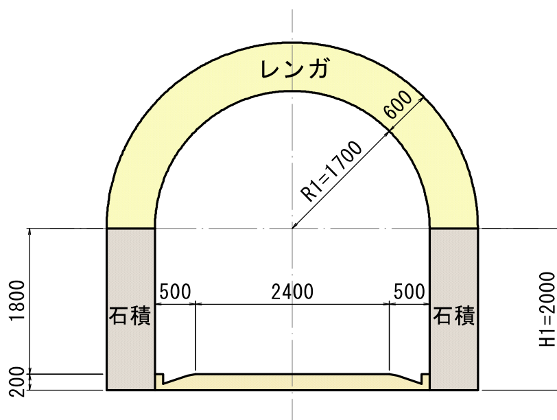
図 1.1.2 熊井隧道標準断面図
