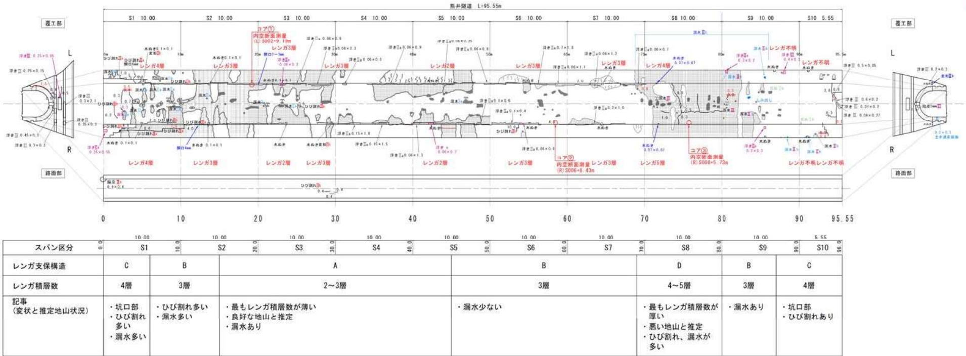
図 1.2.1 熊井隧道の点検調査総括図
