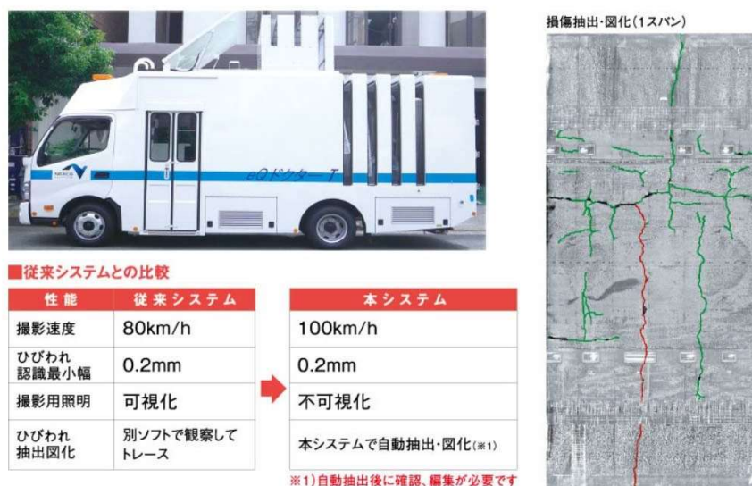
図 2.2.1 トンネル画像取得システムの一例
